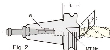
Pull stud draw bolt type.
