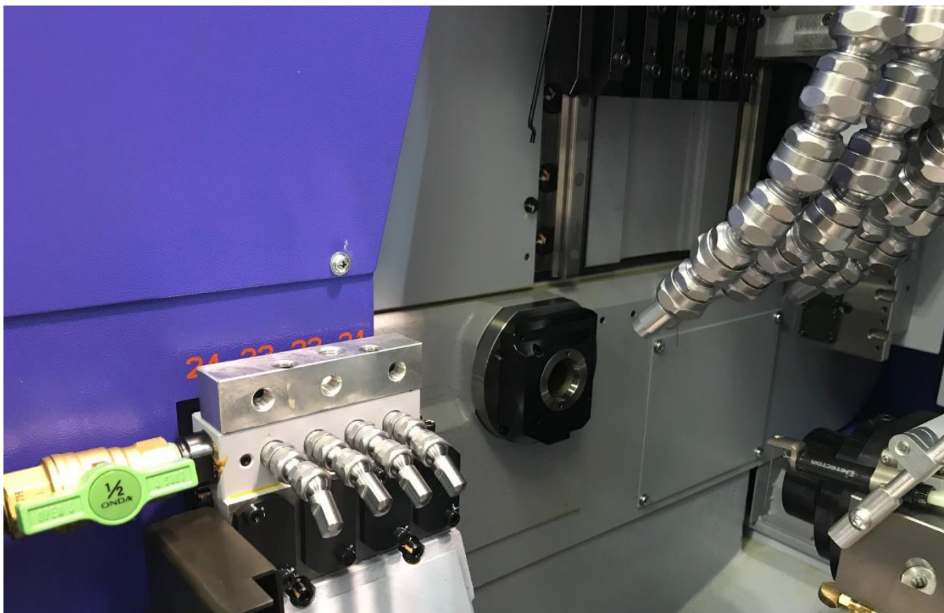
Sistema HECTO para refrigeración en bloque posterior
